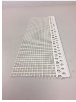
BEB3 - BRICK EDGE BEAD 3MM
